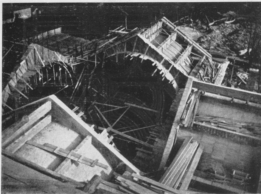
A HOSSZANTI ÉS HARÁNTBOLTOZATOK KÉPE A FEDÉLHÉJAZAT ELHELYEZÉSE ELŐTT
