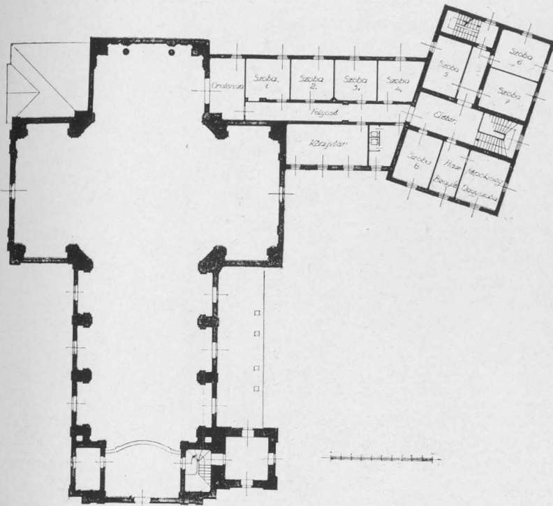
FELSŐ ALAPRAJZ
