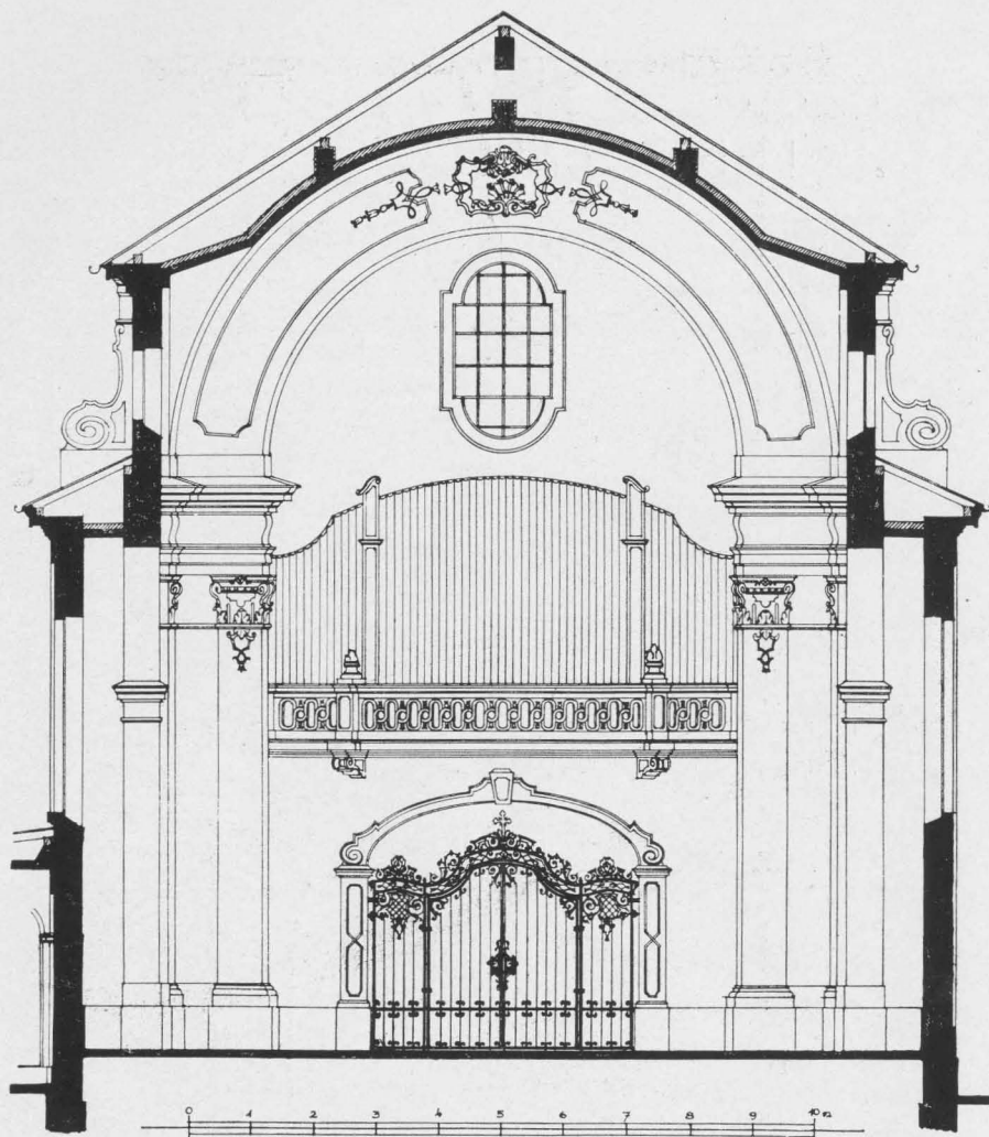
A HOSSZHAJÓ KERESZTMETSZETE, A FŐBEJÁRÓ FELÉ NÉZVE
