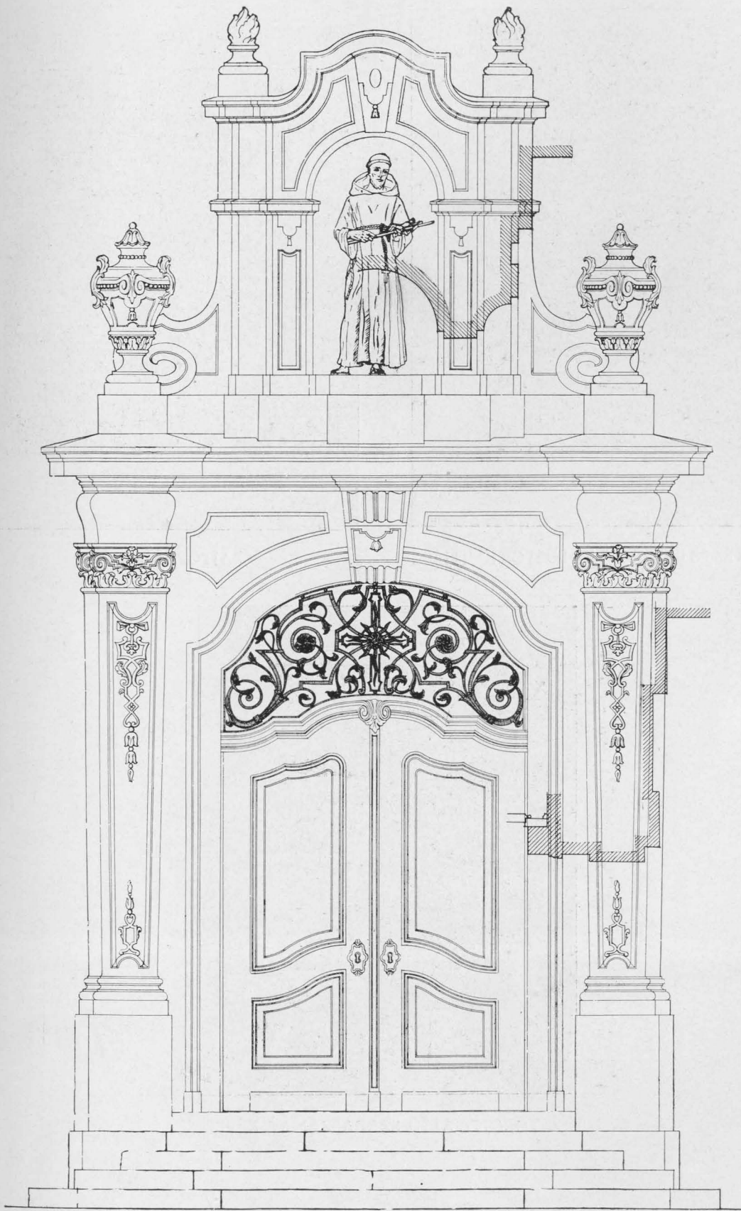
A FŐBEJÁRÓ KAPUZAT ELŐLNÉZETE
