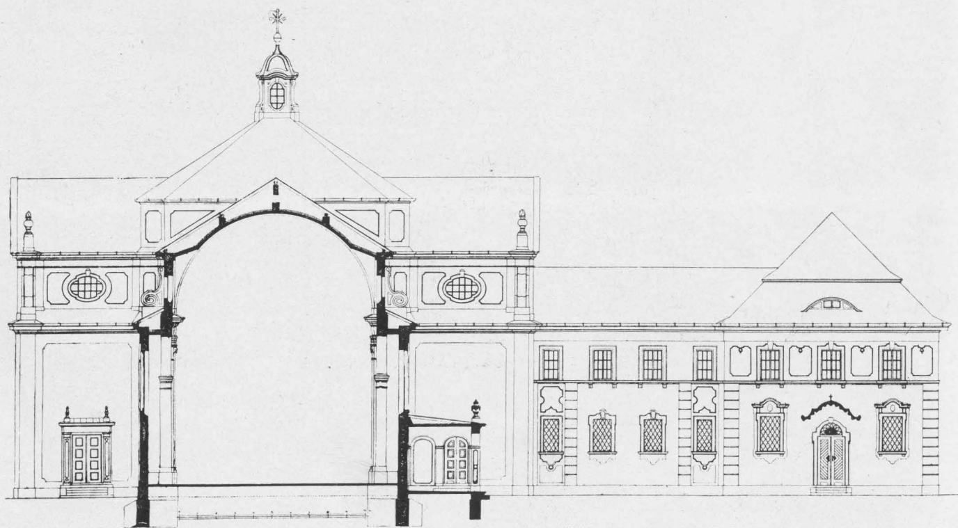
A HOSSZHAJÓ KERESZTMETSZETE, A KOLOSTOR HOMLOKZATÁVAL
