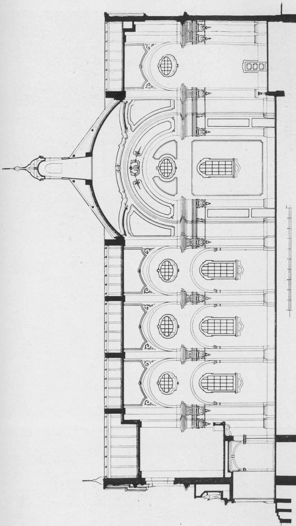
HOSSZMETSZET
