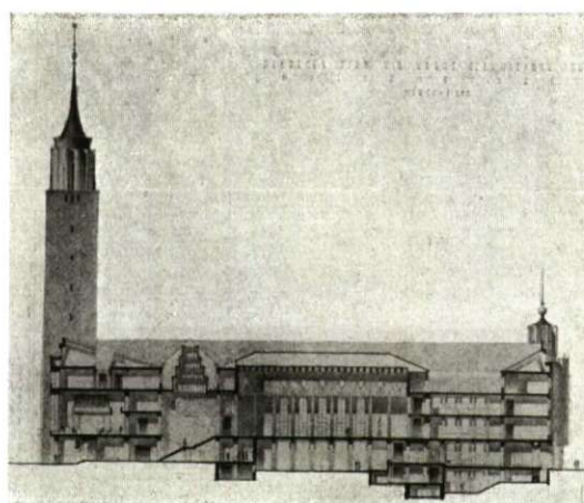
I. DÍJ METSZET GYÖRGYI DÉNES: A DEBRECENI VÁROSHÁZA
