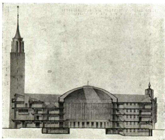
GYÖRGYI DÉNES: A DEBRECENI VÁROSHÁZA AZ ALTERNATÍV TERV METSZETE
