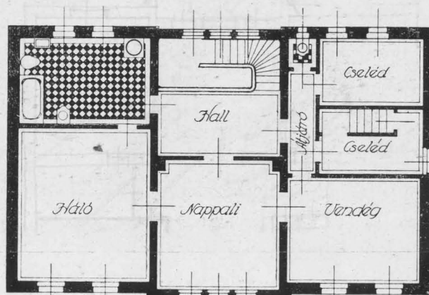
ALAPRAJZOK
