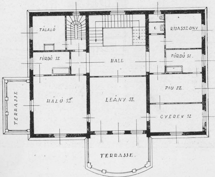
EMELETI ALAPRAJZ
