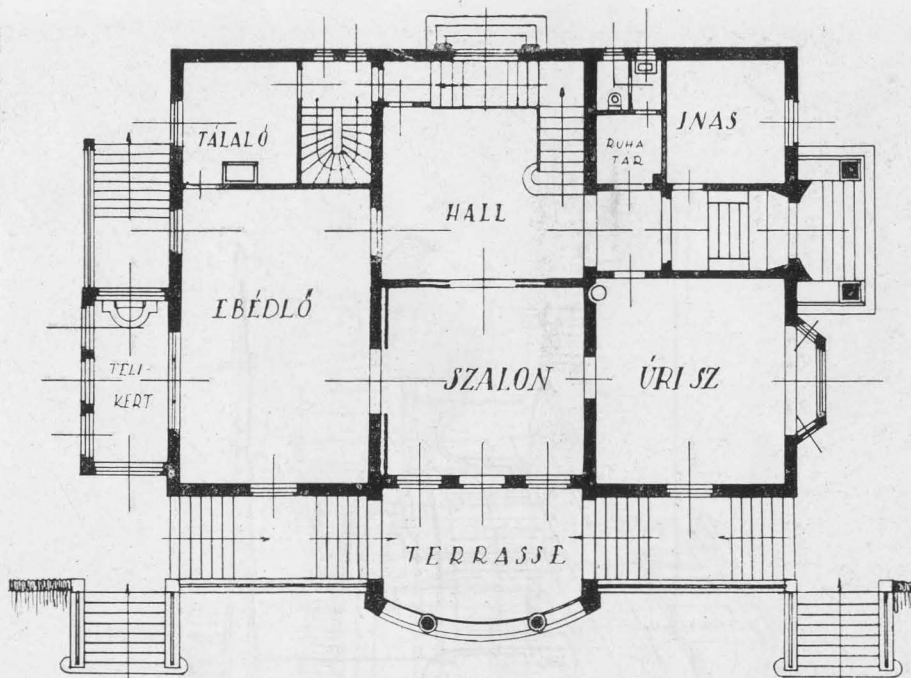
FÖLDSZINTI ALAPRAJZ
