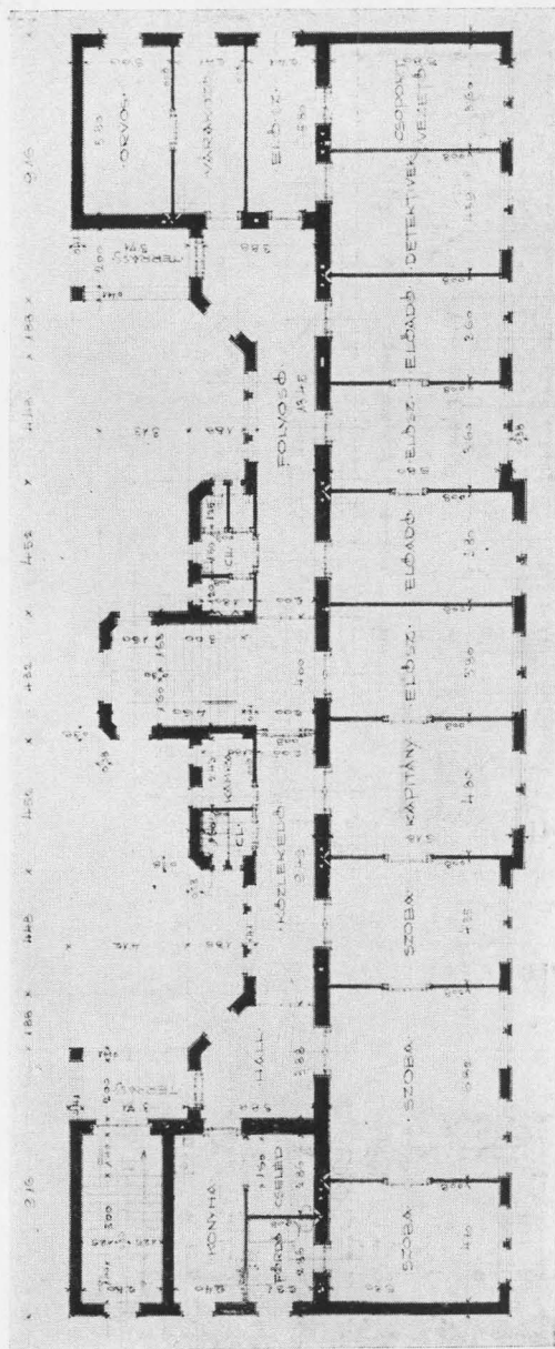
EMELETI ALAPRAJZ
