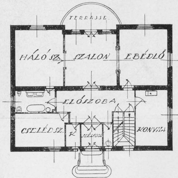
ALAPRAJZ GELLÉRTHEGYI SCHEFARCSIK-VILLA
