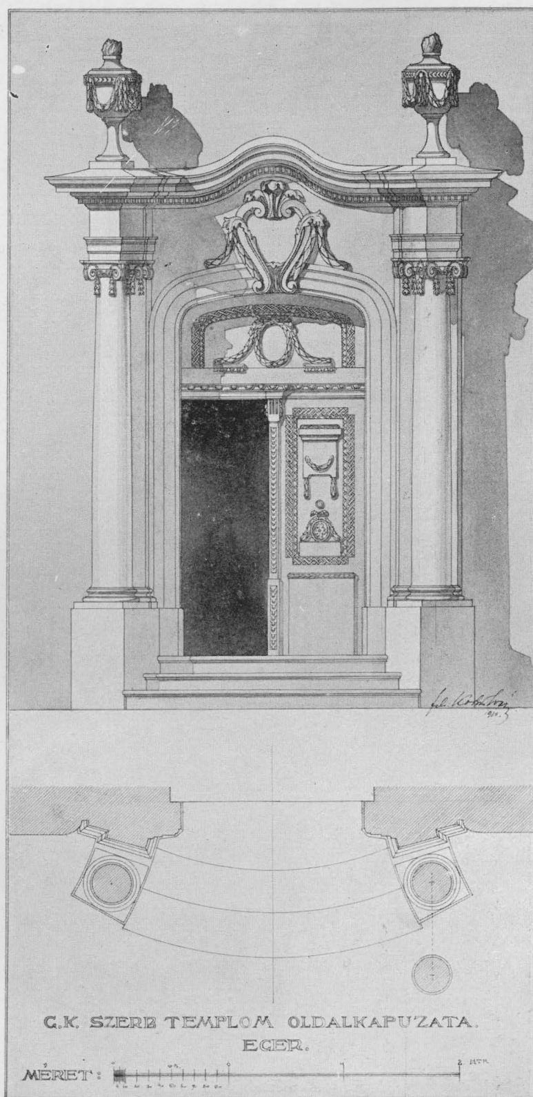
AZ EGRI GÖRÖGKELETI TEMPLOM BEJÁRATA
