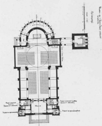
A FERENC JÓZSEF JUBILEUMI TEMPLOM PÁLYATERVE
