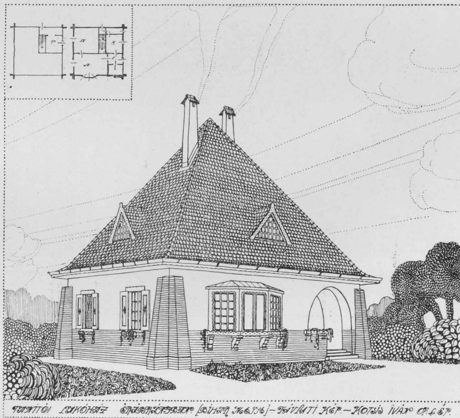
TANÍTÓI LAK ÉRÁBRÁNYBAN
