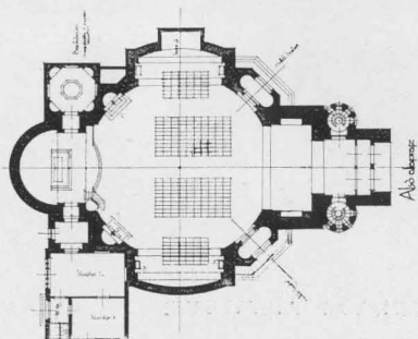
AZ ARADI RÓM. KAT. TEMPLOM DÍSZAZOTT PÁLYATERVE
