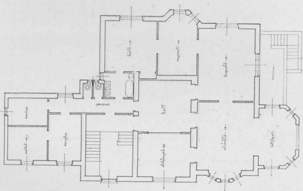
LAKÓHÁZ A GELLÉRTHEGYEN
