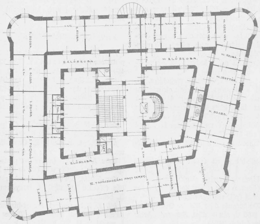
I. EM. ALPRAJZ.
