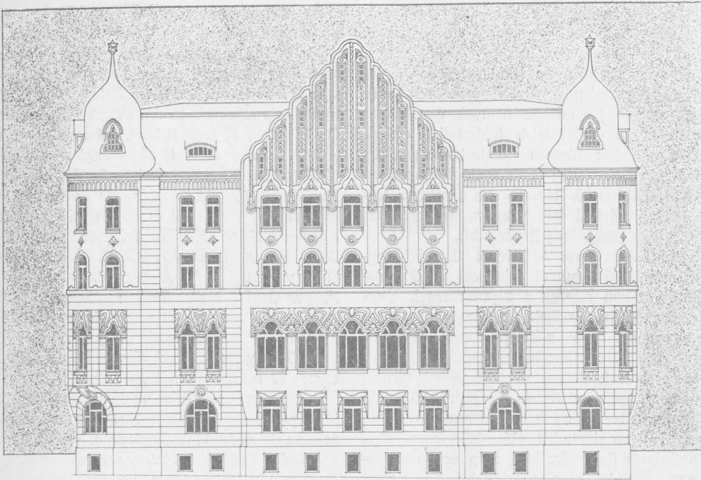
FŐHOMLOKZAT.
