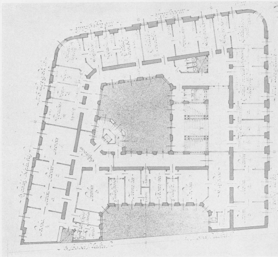
III. EM. ALAPRAJZ. BALINT ZOLTÁN ÉS JÁMBOR LAJOS, BUDAPEST.
