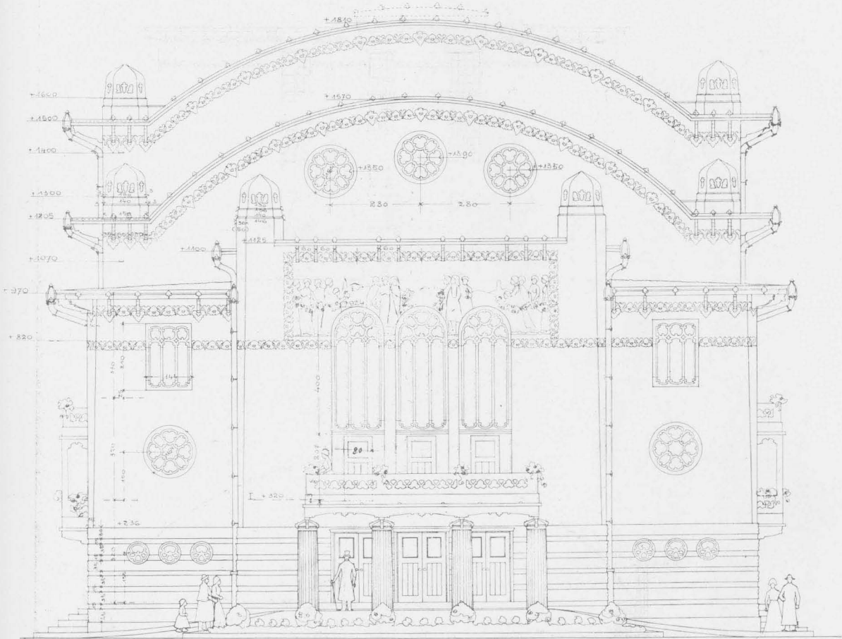
FŐHOMLOKZAT.
