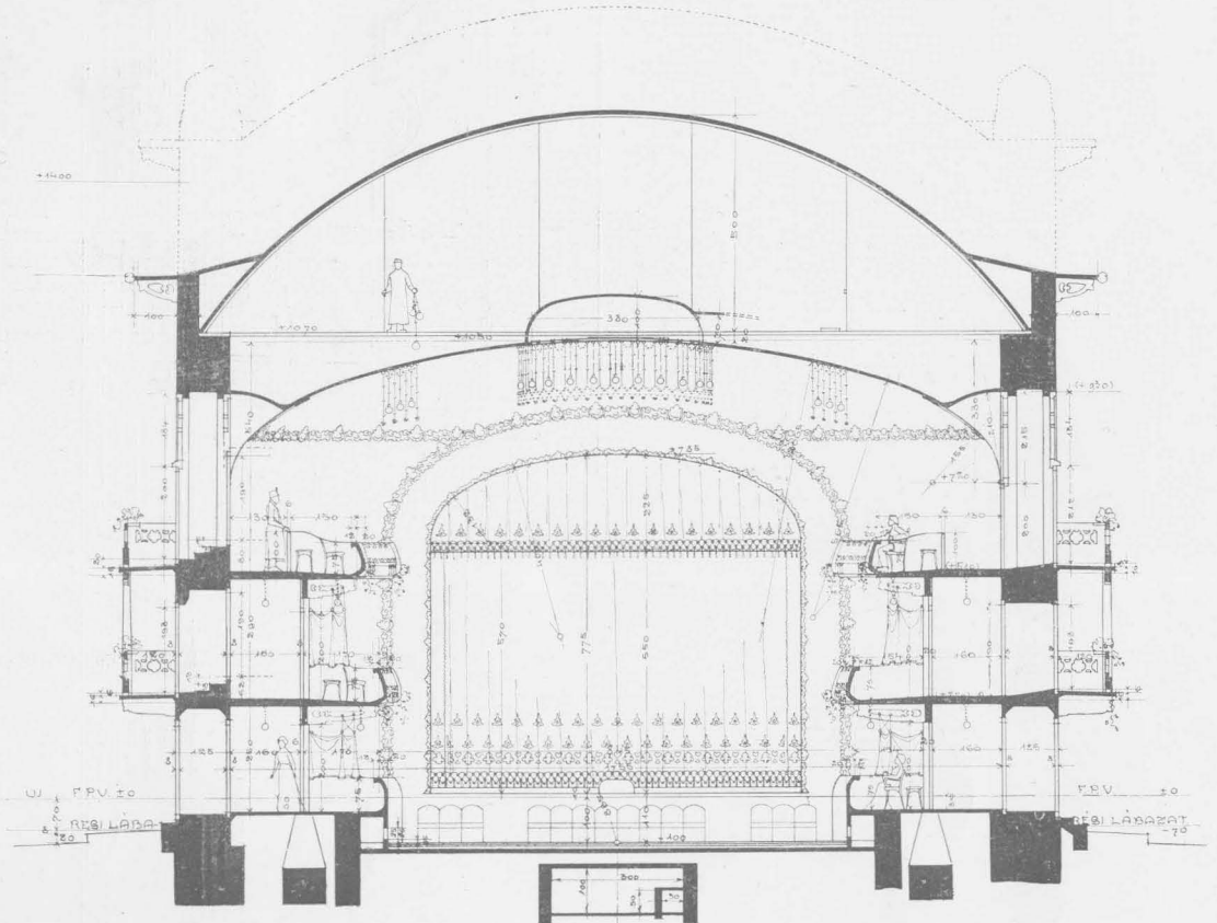
METSZET.
