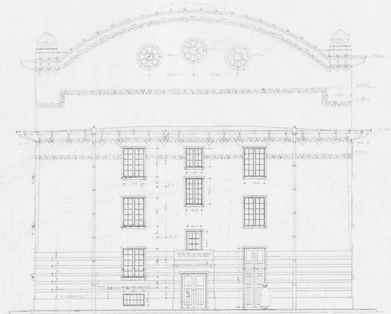
HÁTSÓ HOMLOKZAT.
