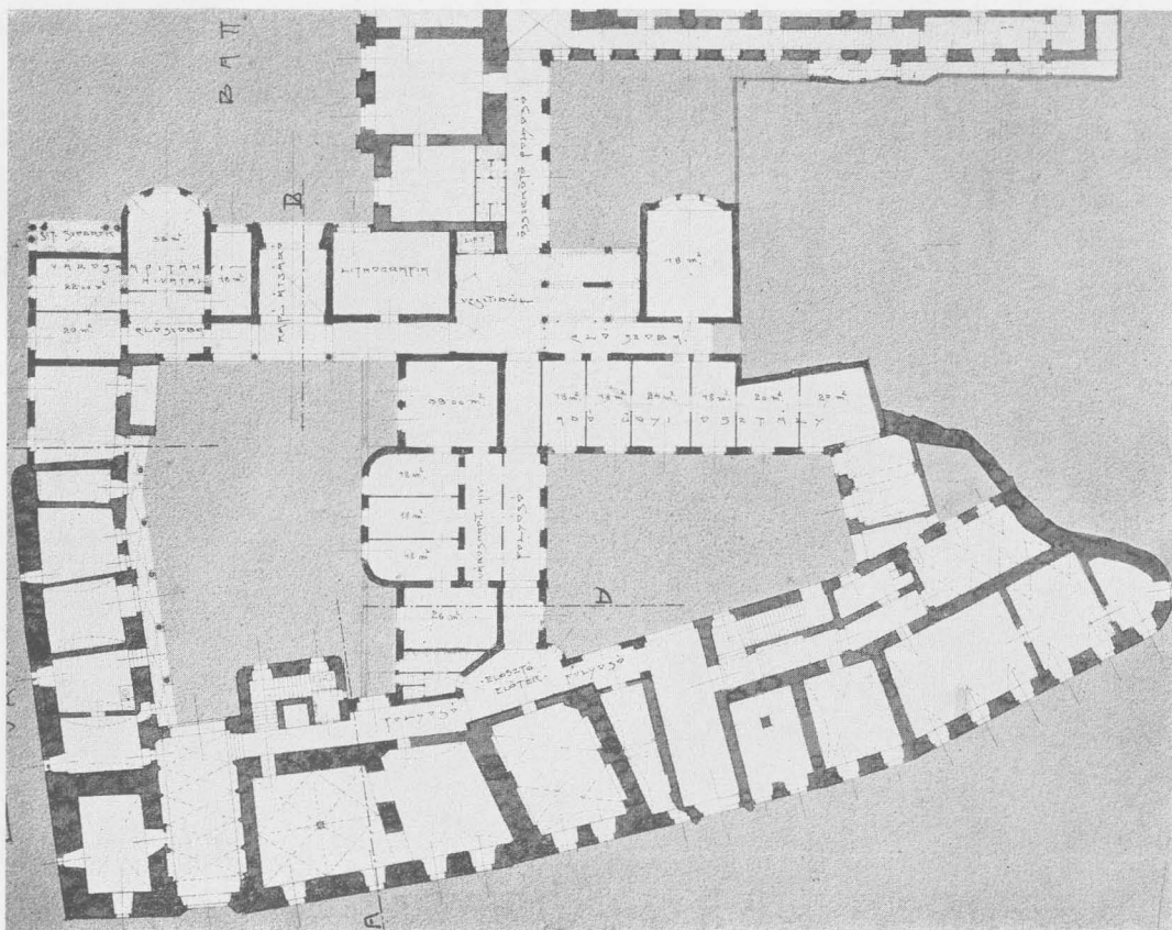
FÖLDSZINTI ALAPRAJZ.
