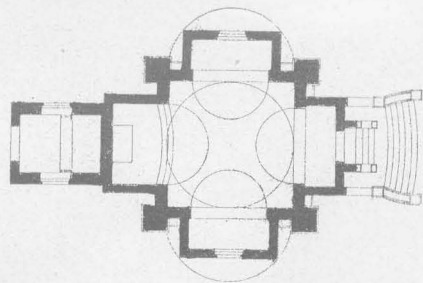
A kápolna alaprajza.
