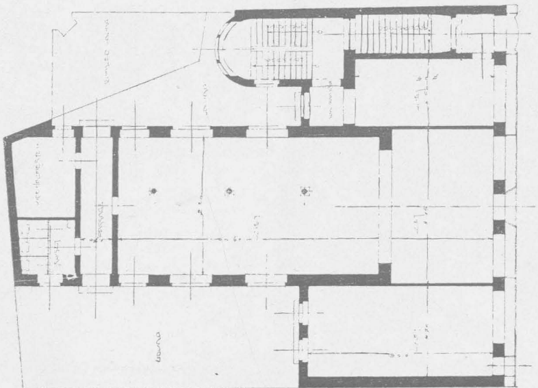
Földszinti alaprajz.
