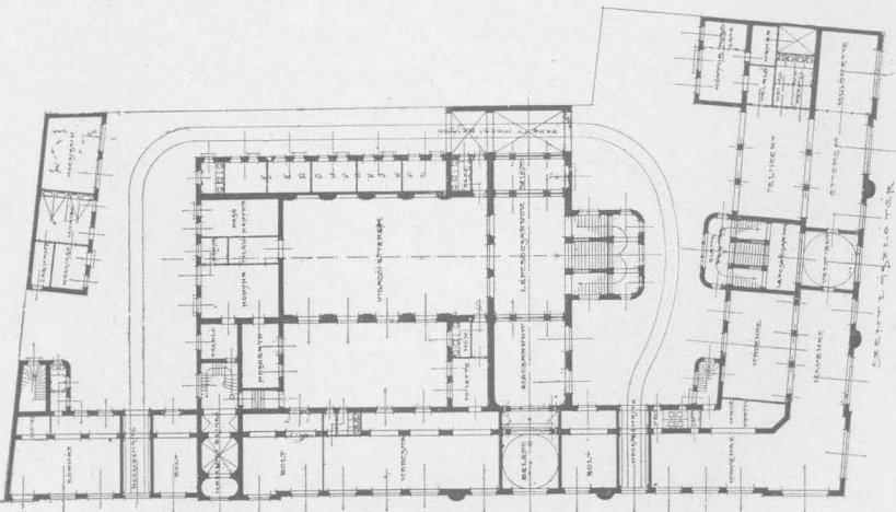
Földszinti alaprajz.
