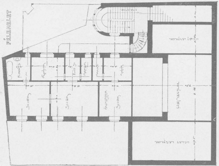
Félemeleti alaprajz.
