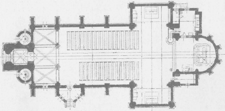
Alaprajz.
