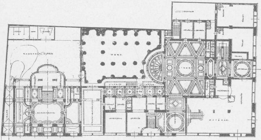
Földszinti alaprajz.
