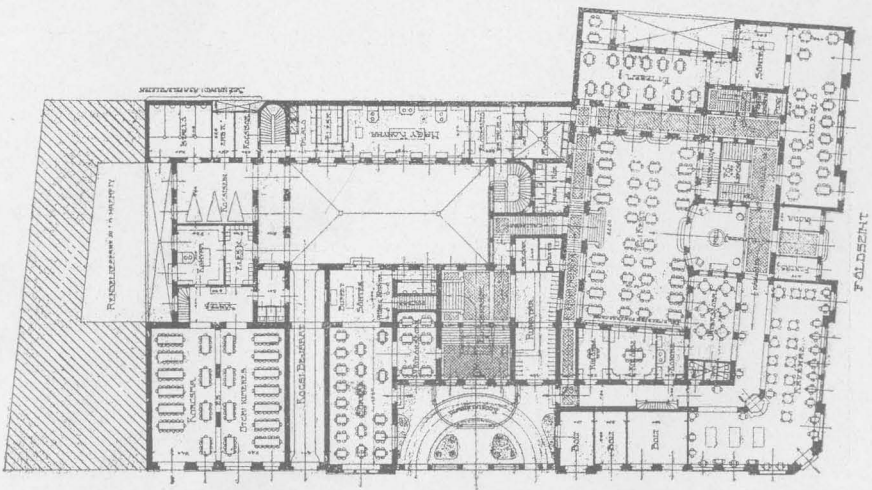
Földszinti alaprajz.
