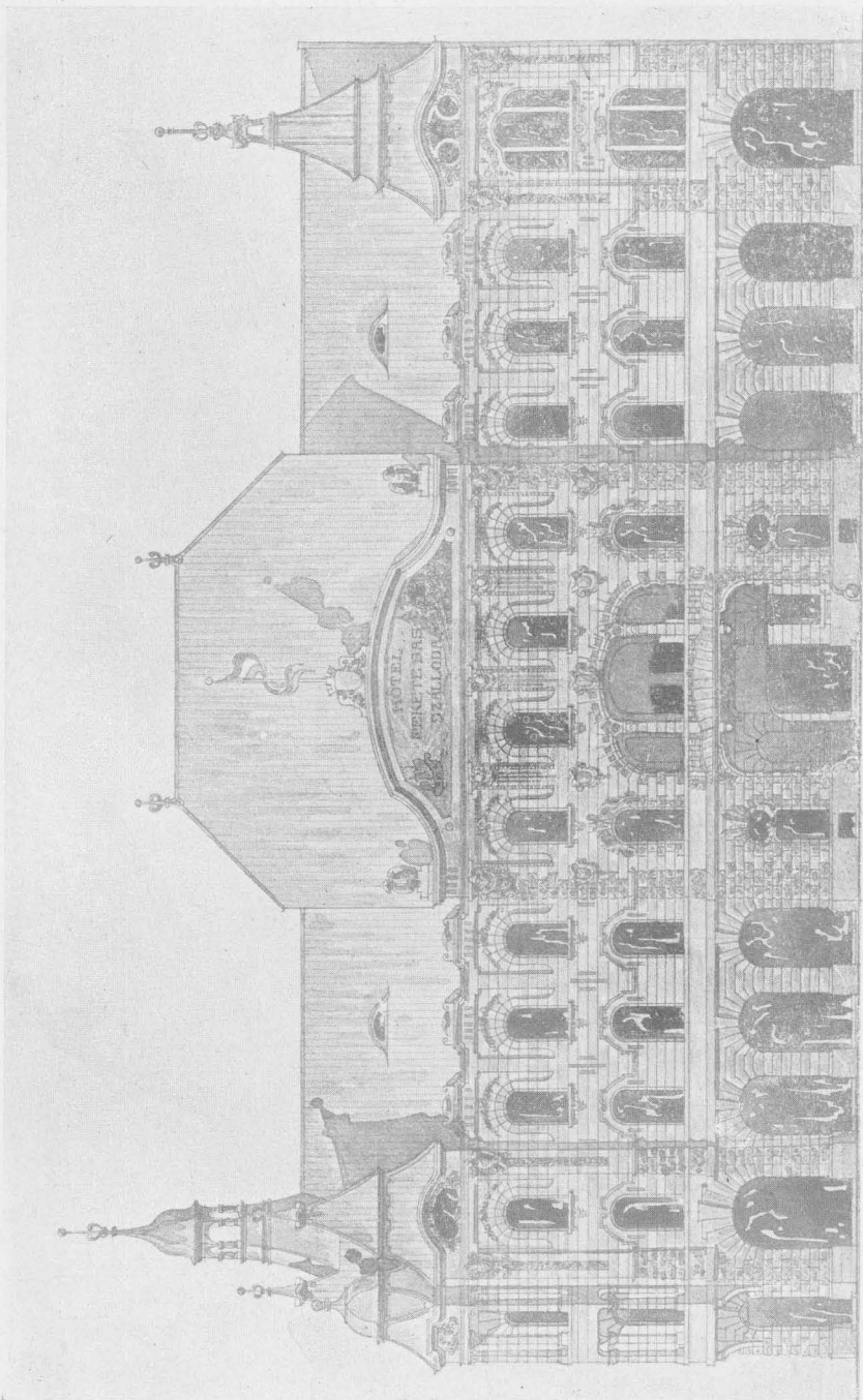
Főhomlokzat.
