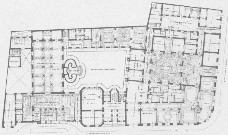
Földszinti alaprajz.
