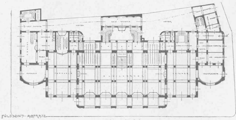
Földszinti alaprajz.
