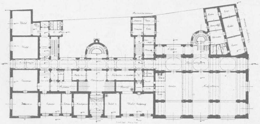
Földszinti alaprajz.
