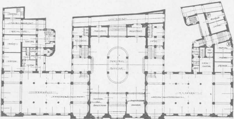
Földszinti alaprajz
