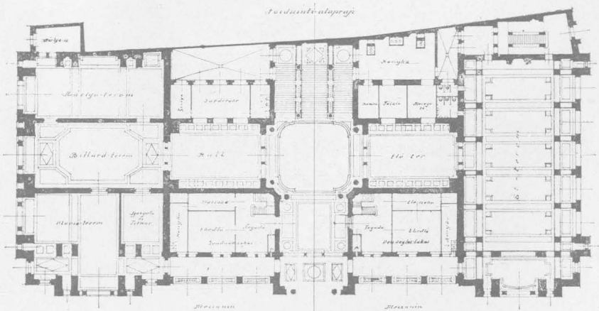
Földszinti alaprajz.
