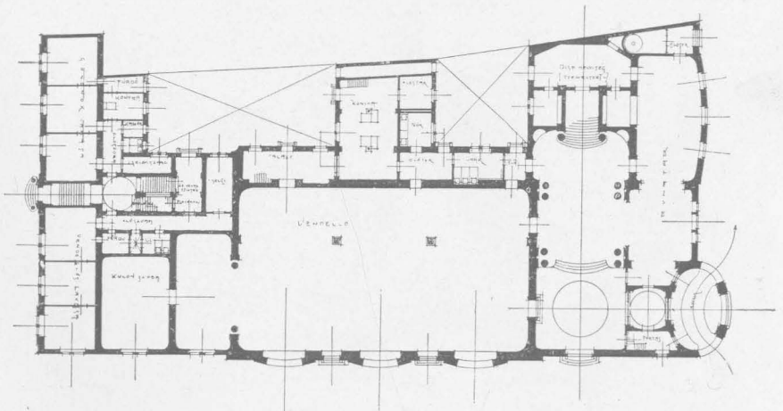
Földszinti alaprajz.
