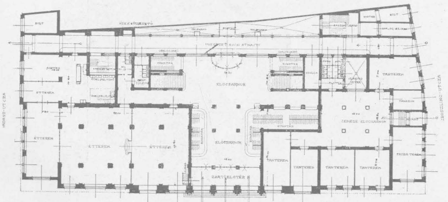
Földszinti alaprajz.
