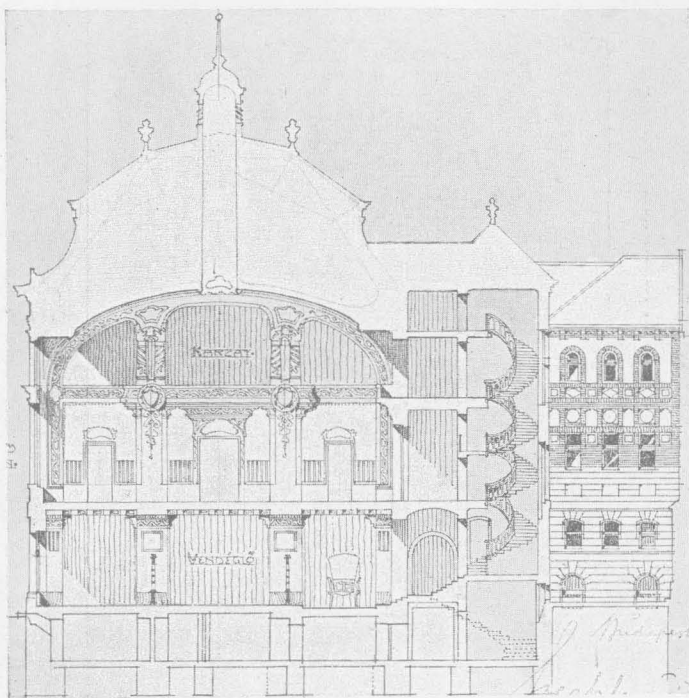
Metszet.
