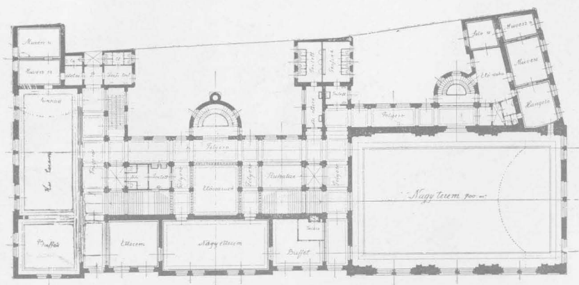
I. em. alaprajz.
