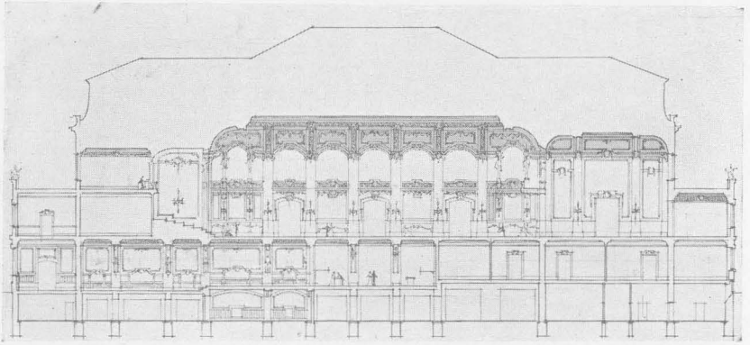
Metszet.
