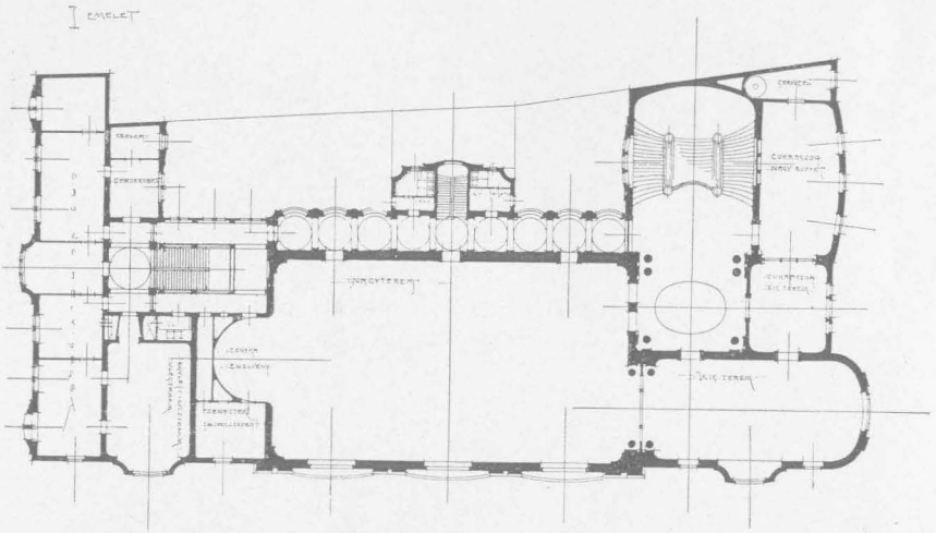
I. em. alaprajz.
