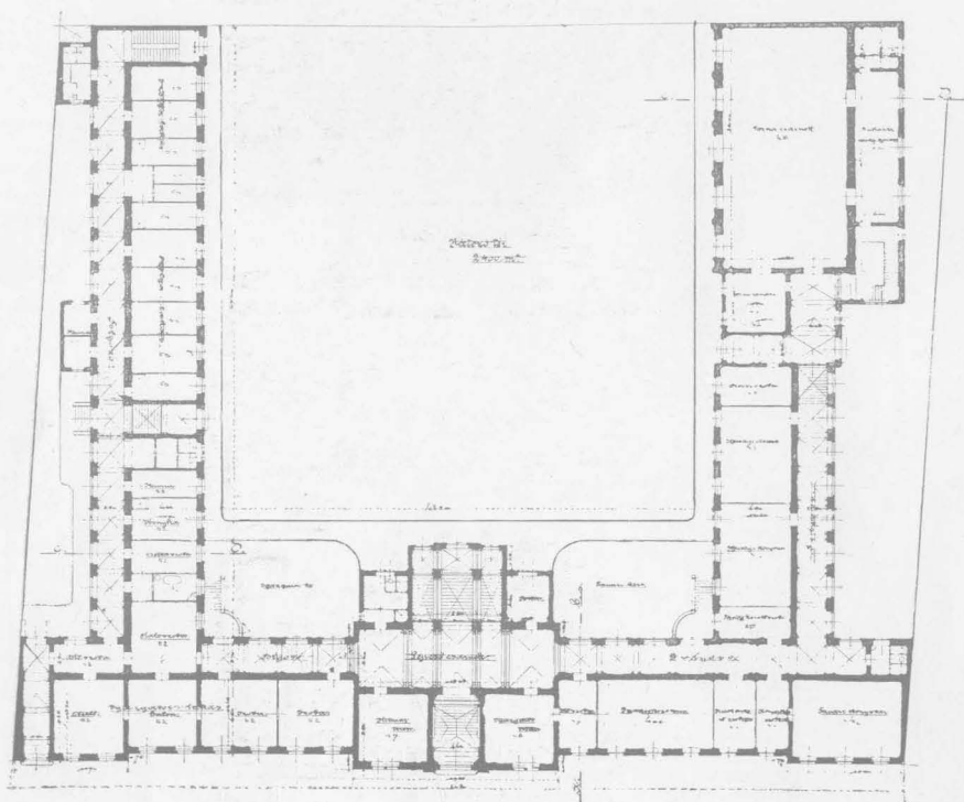
Földszinti alaprajz.
