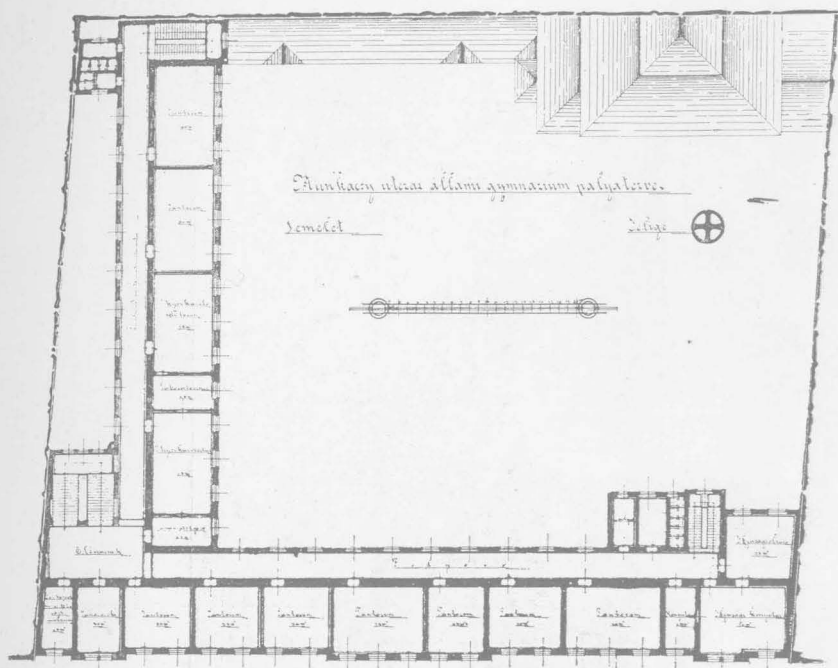
I. em. alaprajz.
