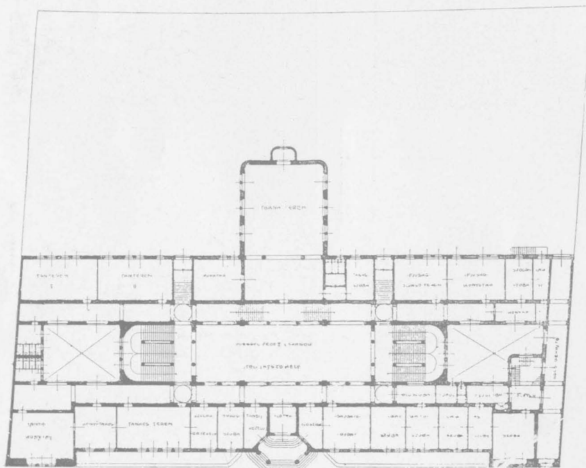
Földszinti alaprajz.
