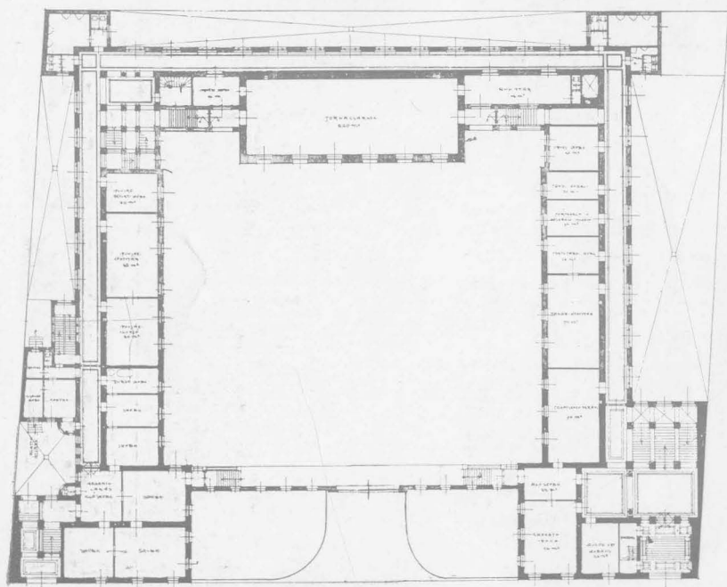
Földszinti alaprajz.
