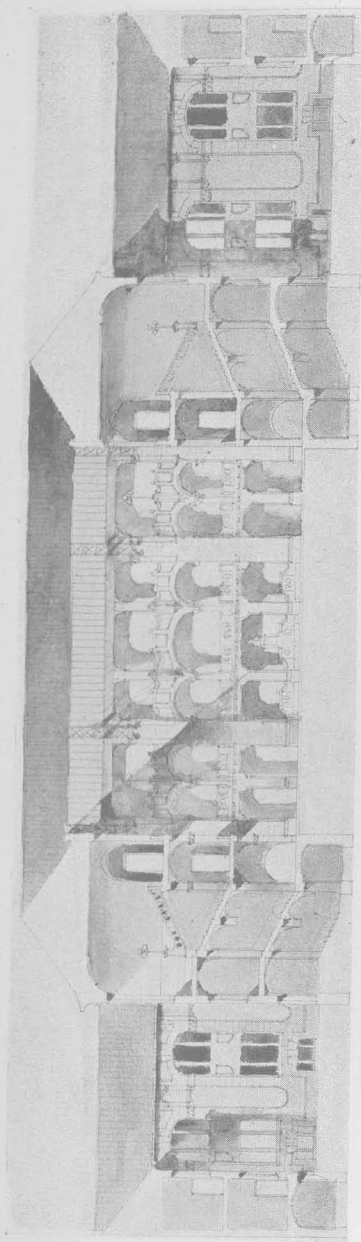
Hosszmetszet.
