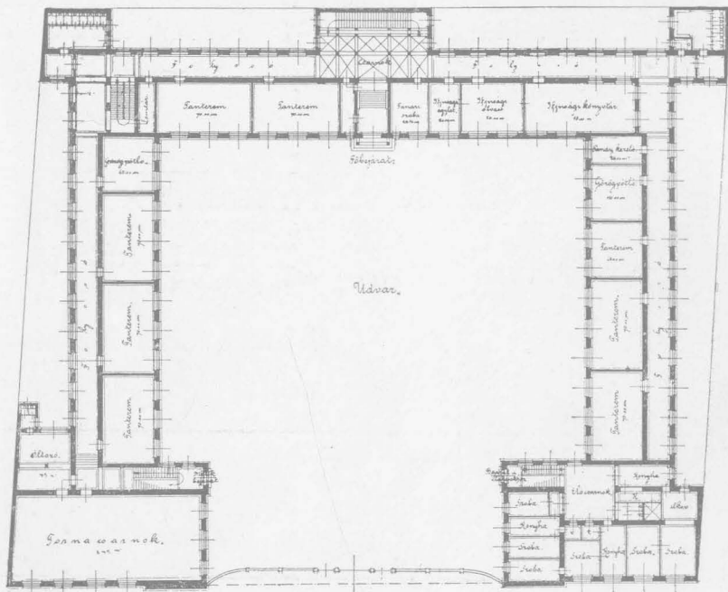
Földszinti alaprajz.
