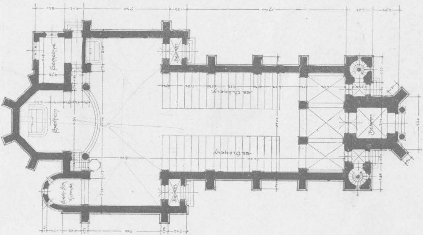
Földszinti alaprajz.
