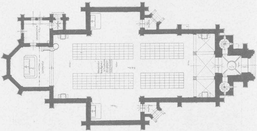
Földszinti alaprajz.
