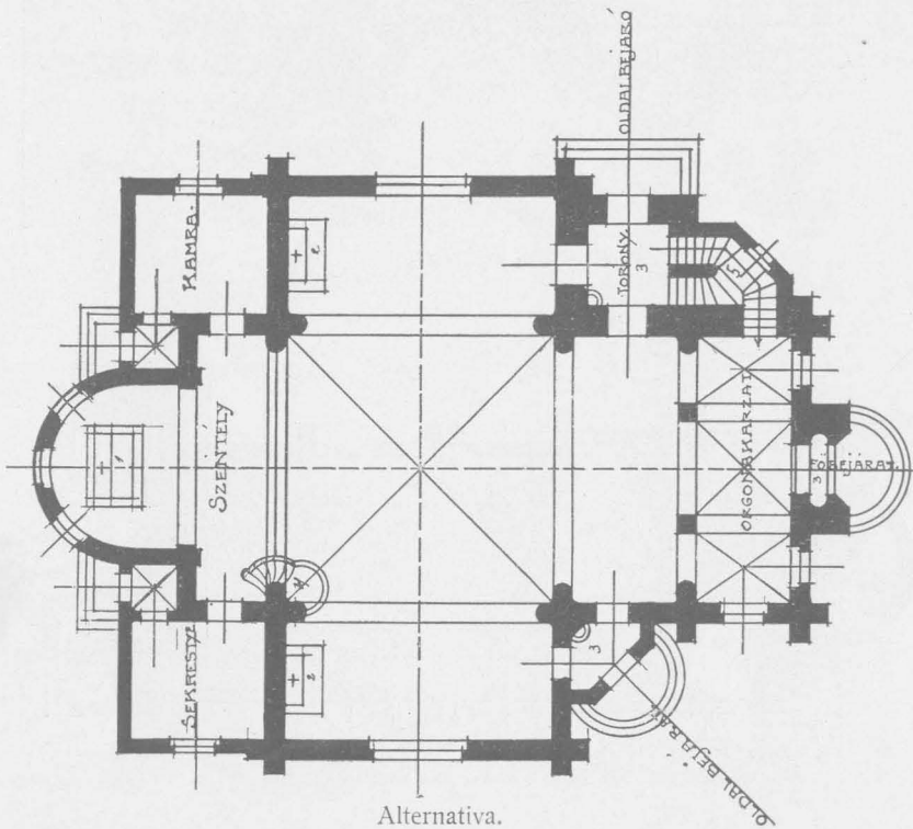
Földszinti alaprajz.
