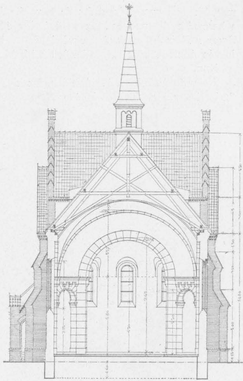
Metszet.
