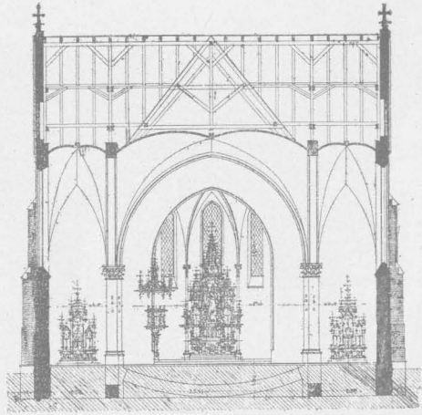
Metszet.
