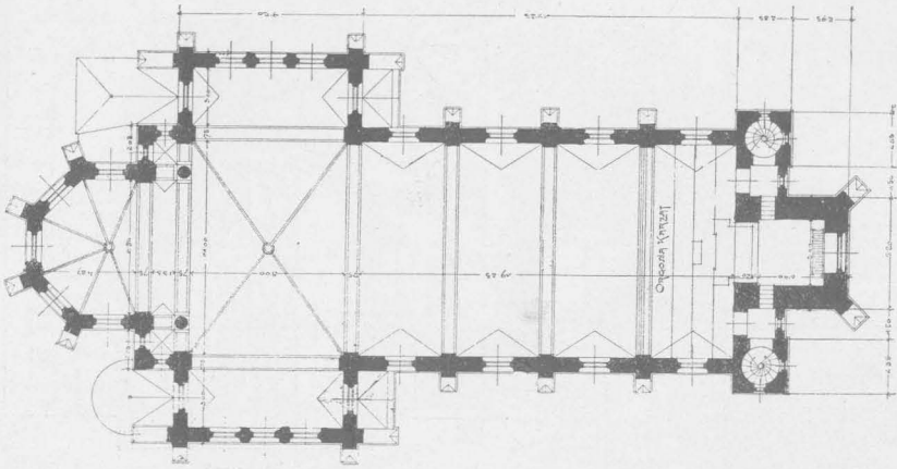
Emeleti alaprajz.
