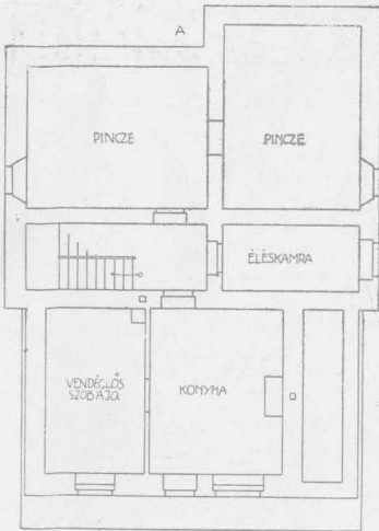
Földszinti alaprajz.
