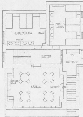
Emeleti alaprajz.
