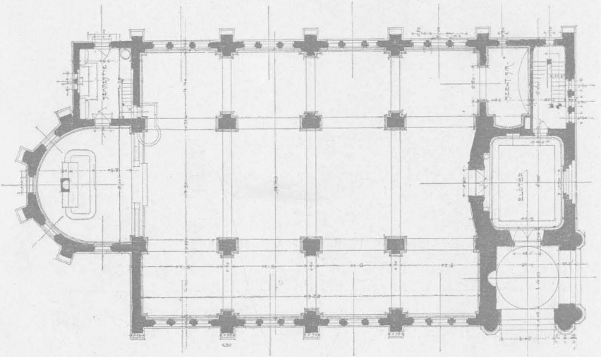
Földszinti alaprajz.
