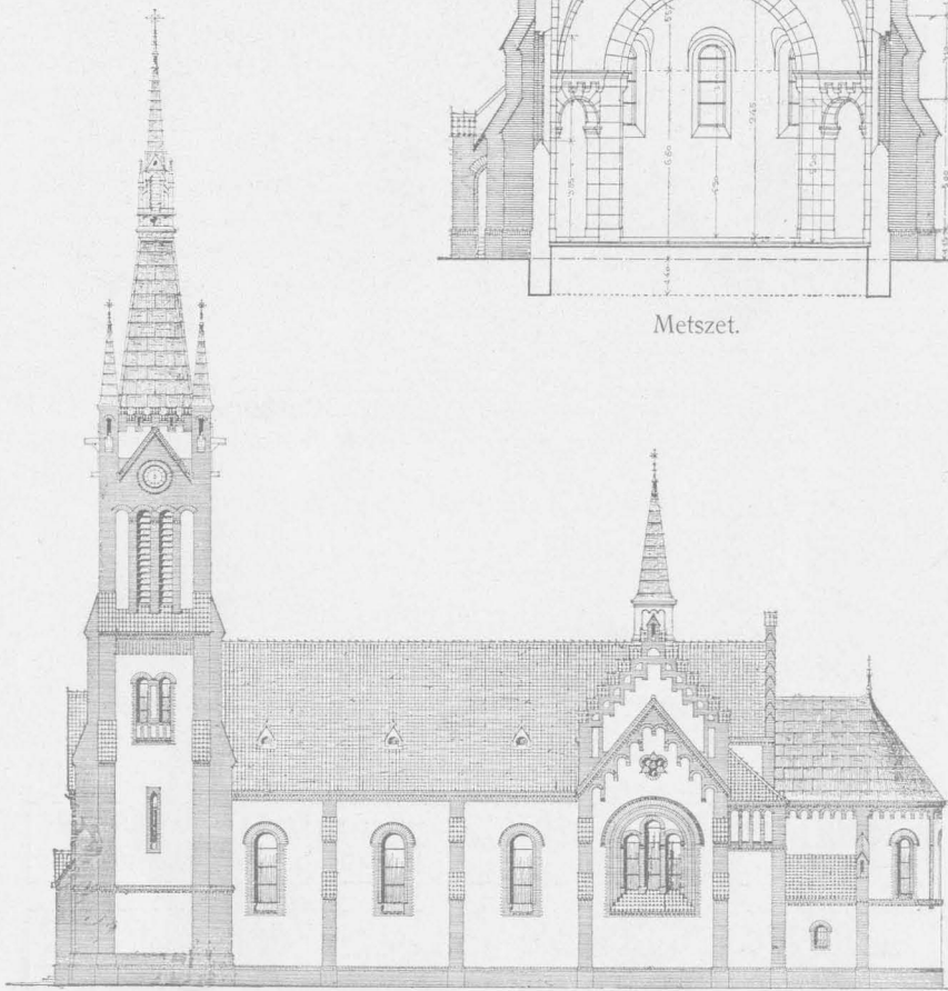
Oldalhomlokzat.
