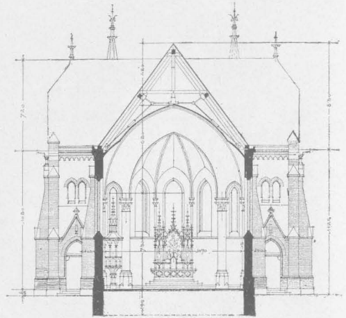
Metszet.
