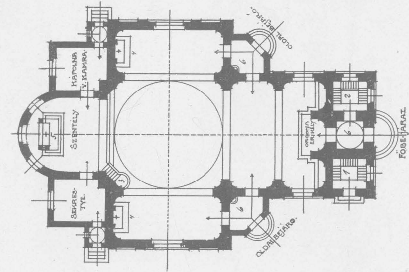
Földszinti alaprajz.
