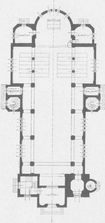
Földszinti alaprajz
