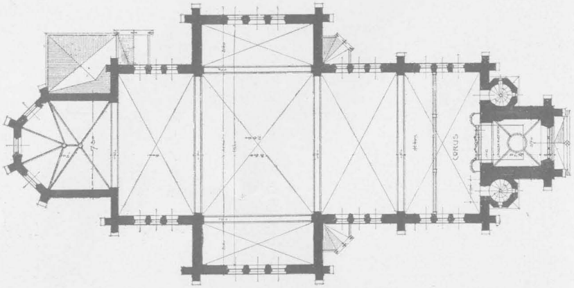
Emeleti alaprajz.
