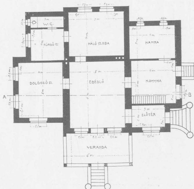
6. sz. — Jelige: Si duo faciunt idem. Fáy László és Kürthy György, Budapest. Megdicsért terv.
