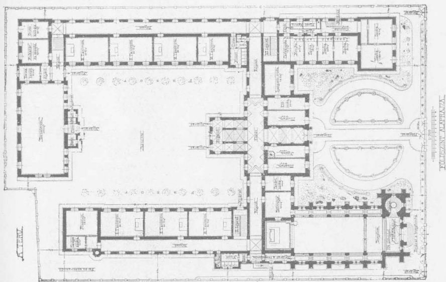
Földszinti alaprajz.
