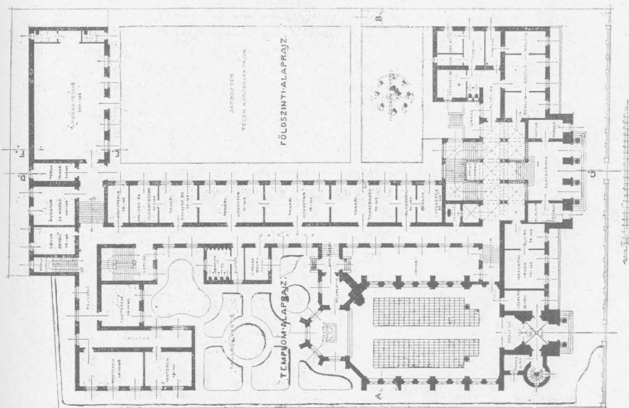
Földszinti alaprajz.
