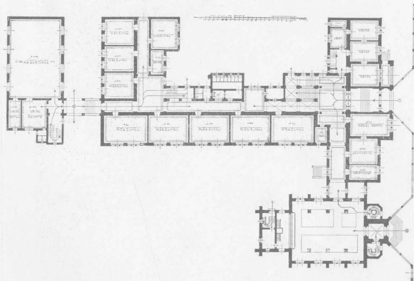
Földszinti alaprajz.
