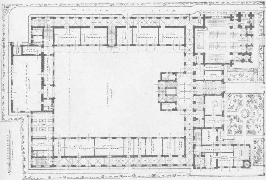
Földszinti alaprajz.
