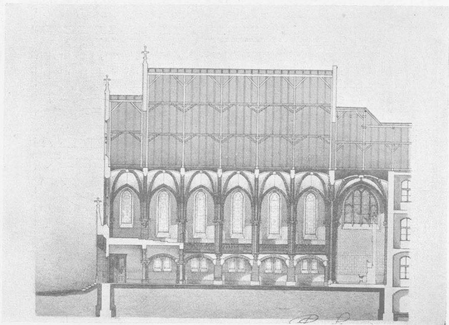
Hosszmetszet.
