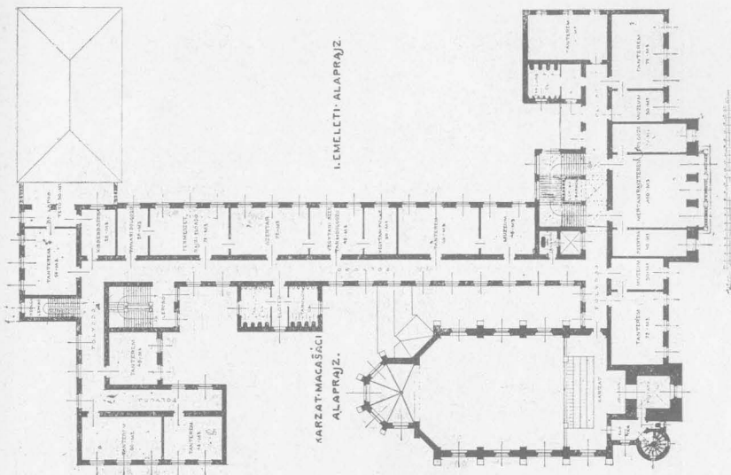
I. emeleti alaprajz.
