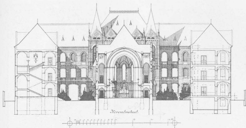
Metszet.
