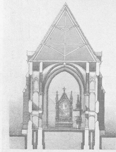
Keresztmetszet.
