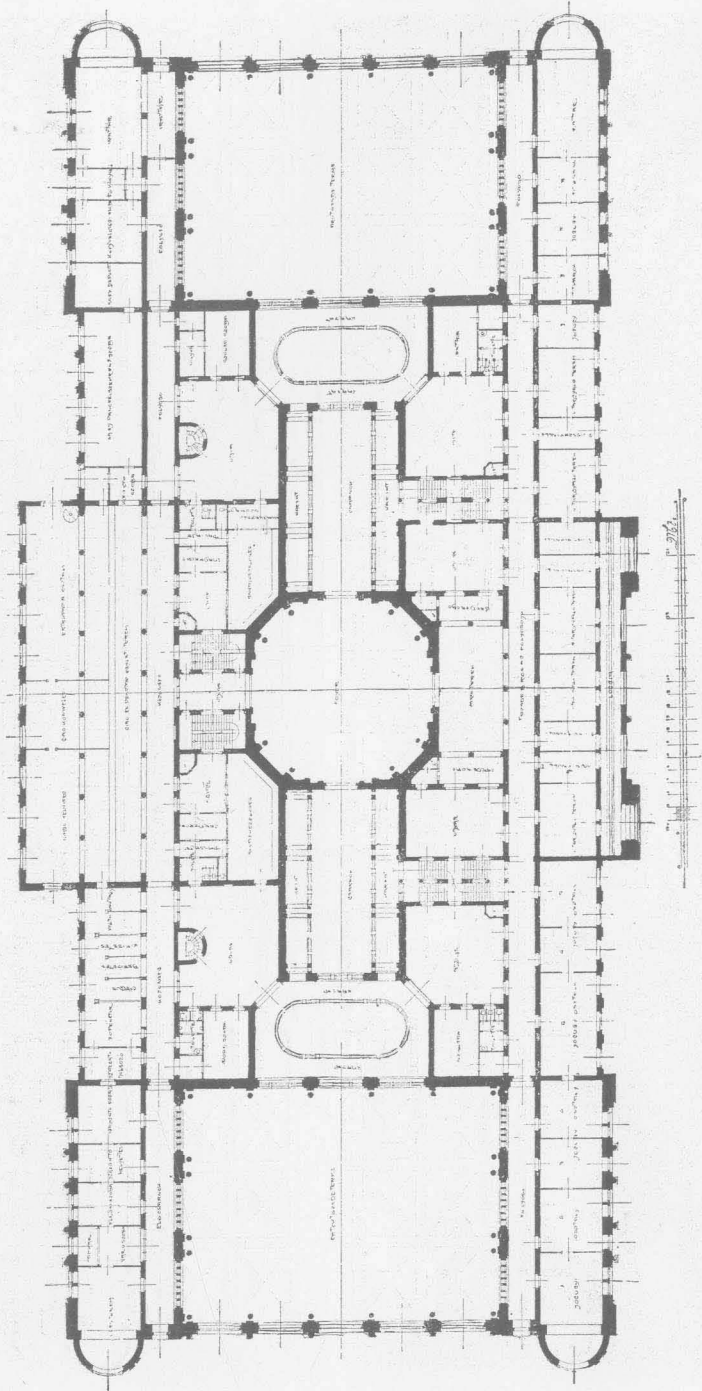
I. emeleti alaprajz.
