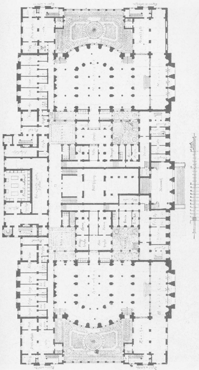
Földszinti alaprajz.
