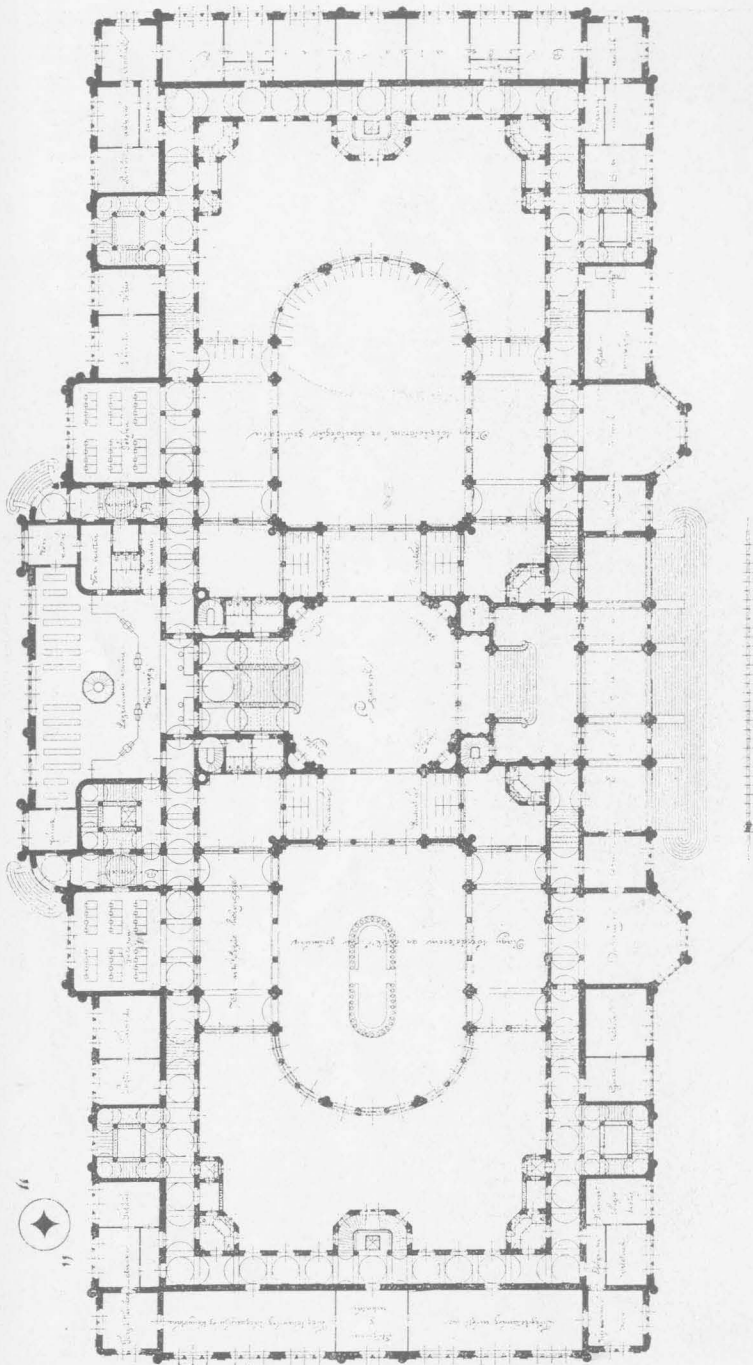
Magas-földszinti alaprajz.
