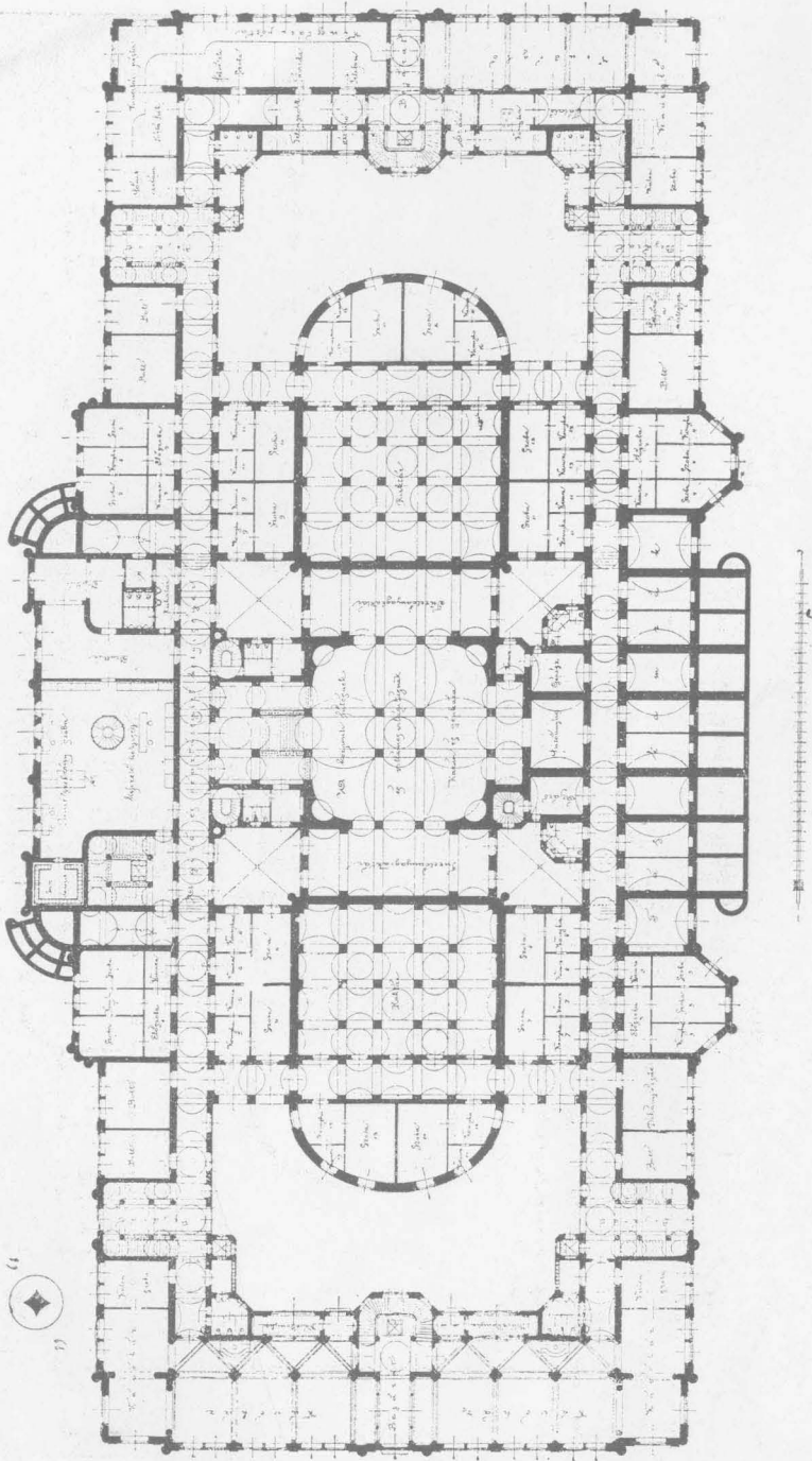
Földszinti alaprajz.
